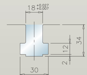
V-1600 T-Slot dimensions
