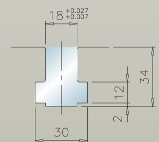
V-2000 T-Slot dimensions
